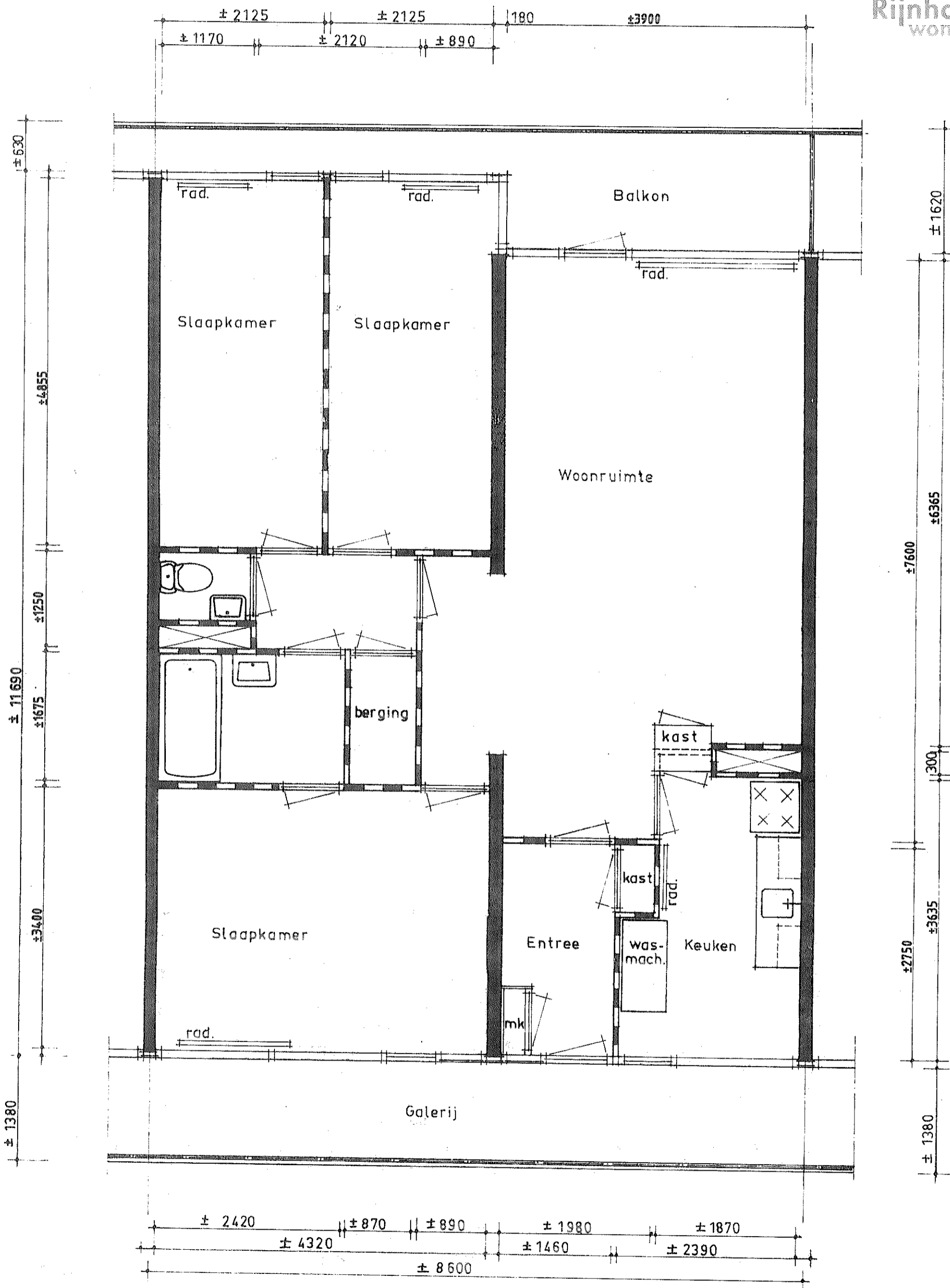
Plattegrond 1:50
